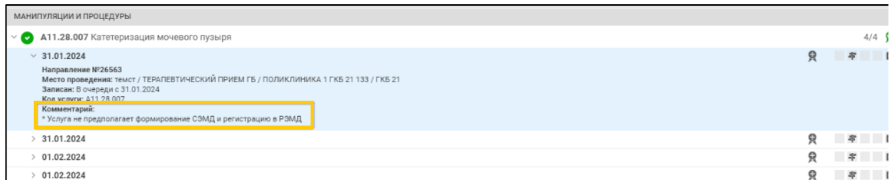
Рисунок 12 – Сообщение Системы
