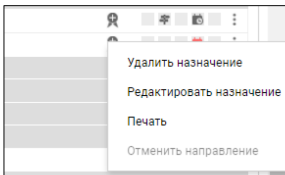
Рисунок 13 – Меню действий
